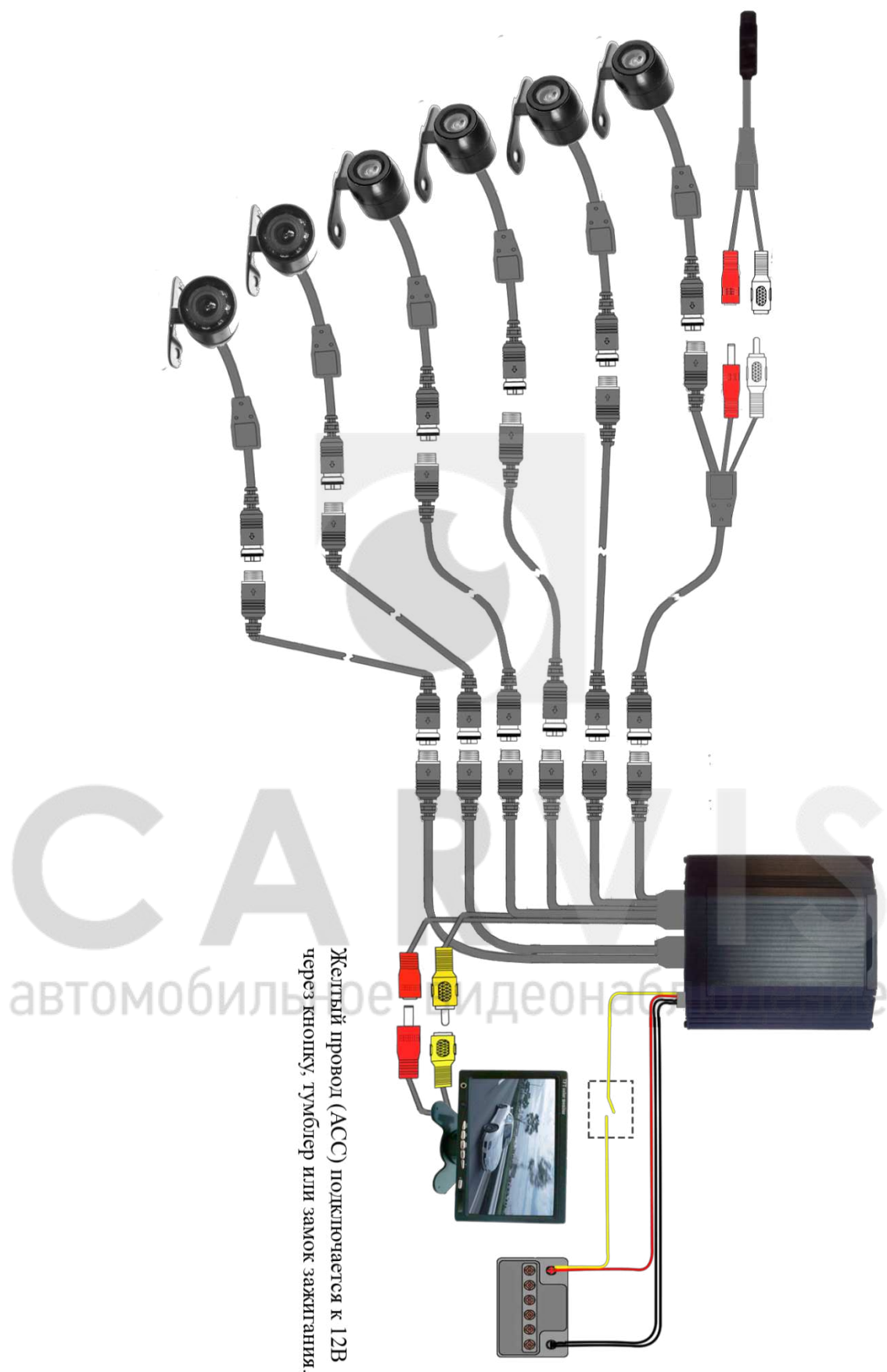
Схема подключения комплекта видеонаблюдения для автошкол 6-ти канального.
